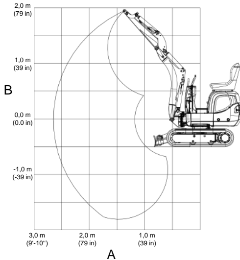
Abb. 1: Hubkrafttabelle 803
