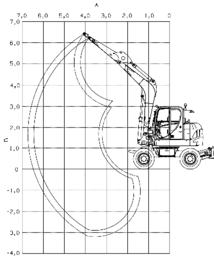
Abb. 1: Hubkrafttabelle EW100 - Monoausleger
