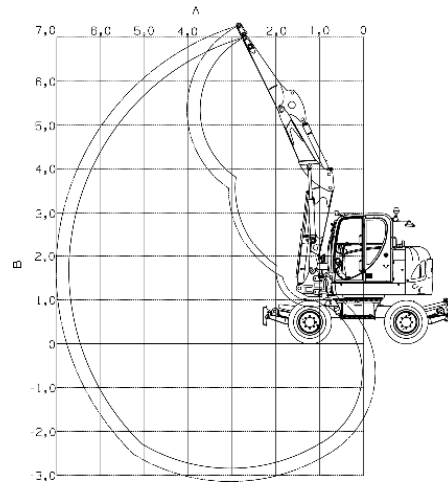
Abb. 2: Hubkrafttabelle EW100 - Verstellausleger
